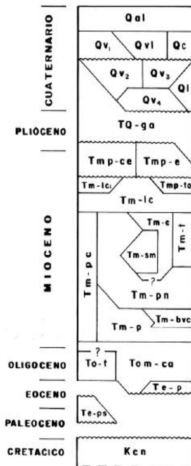
Fig. 2: Columna estratigráfica. Complejo de Nicoya (Ken), Fm. Punta Serrucho (Te-ps), Fm. Parritilla (Te-p), Fm. Caragres (Tom-ca), Miembro Tranquerillas (To-t), Fm. Punta Carballo (Tm-pc), Fm. Pacacua (Tm-p), Brechas verdes Coyolar (Tm-bvc), Fm. Peña Negra (Tm-pn), Fm. San Miguel (Tm-sm), Fm. Coris (Tm-c), Fm. Turrúcares (Tm-t), Fm. La Cruz (Tm-lc), Depósitos Parálitos de Fm. La Cruz (Tm-lci), Tobitas Ococa (Tmp-to), Intrusivo de Escazú (Tm-p-e), Comubianitas de Escazú (Tm-p-ce), Fm. Grifo Alto (TQ-ga), Fm. Lavas intracañón (Qv4), Fm. Depósitos de Avalancha Ardiente (Qv3), Fm. Orotina (Qv2), Fm. Barva (Qv1), Depósitos lacustres (Ql), Calizas deslizadas (Qc). Lahares y cenizas (Qv1), Depósitos aluviales y coluviales recientes (Qal).
